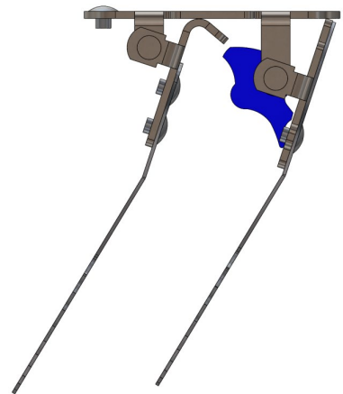
Spjällsystem för TX11 LOCK.
